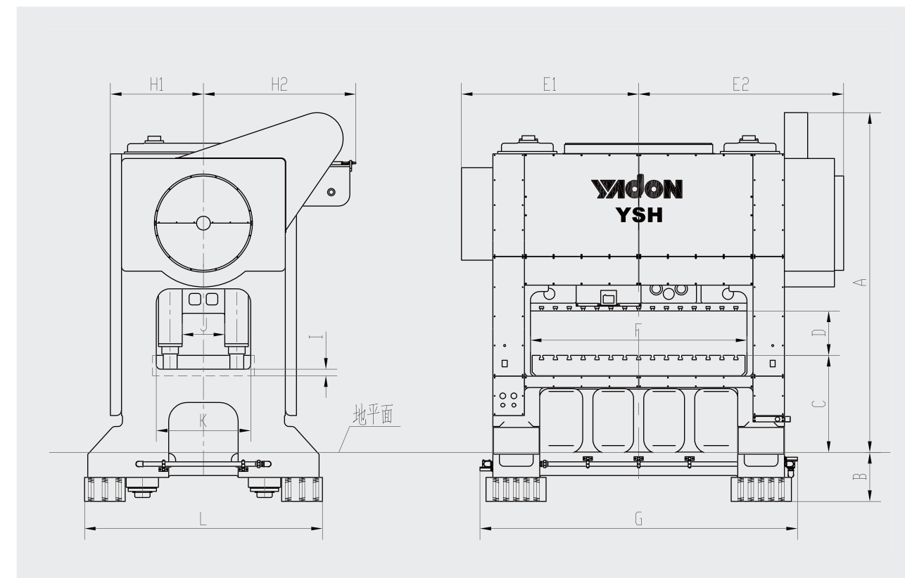
机床外形尺寸图 Outline Size Diagram
